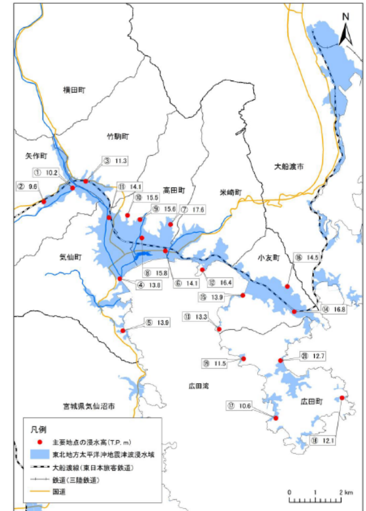
図 1.1 (4) 東北地方太平洋沖地震の津波浸水域と浸水高
